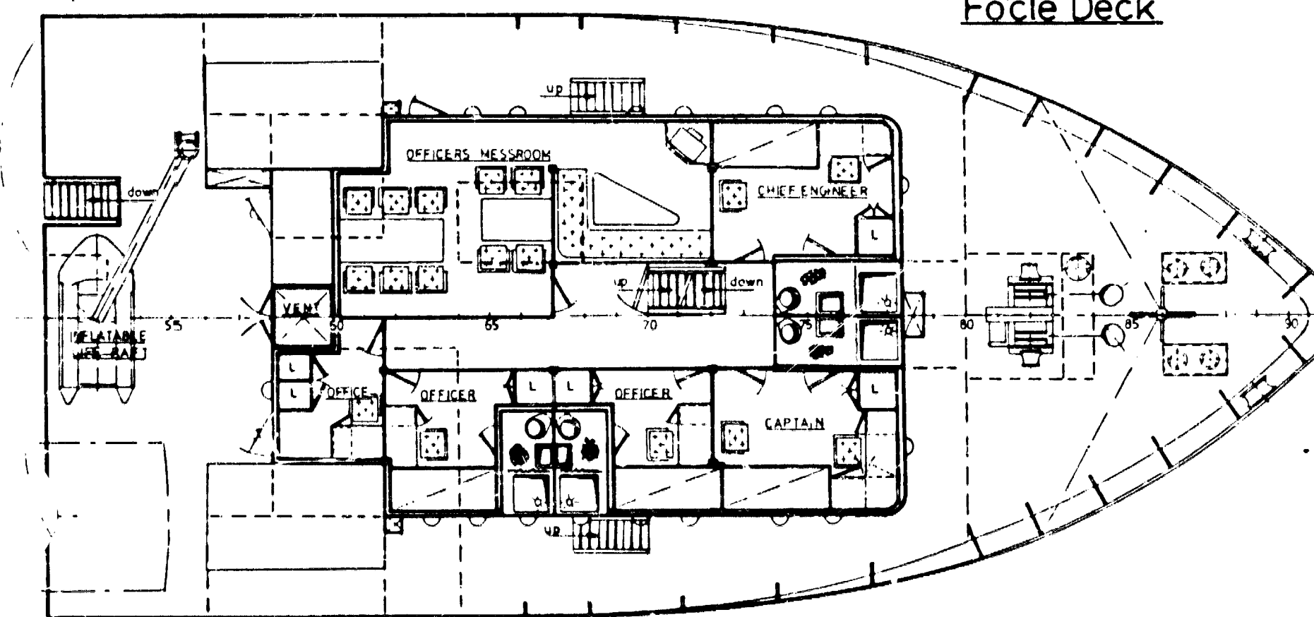
Maindeck
